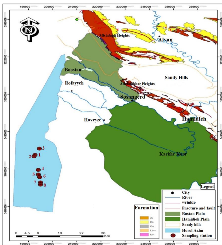
شکل ۲- نقشه زمین شناسی منطقه مورد مطالعه Fig. 2. Geological map of the studied area
