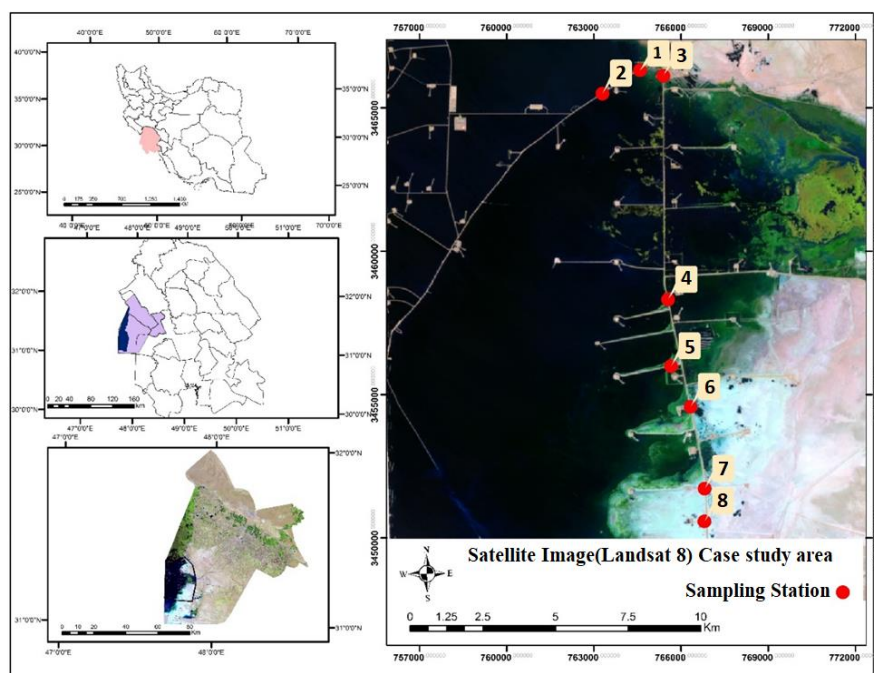
شکل ۱- منطقه مورد مطالعه (امتداد شمال به جنوب بخش شرقی تالاب) Fig. 1. Area of study (The north to south extension of the eastern part of the wetland)
