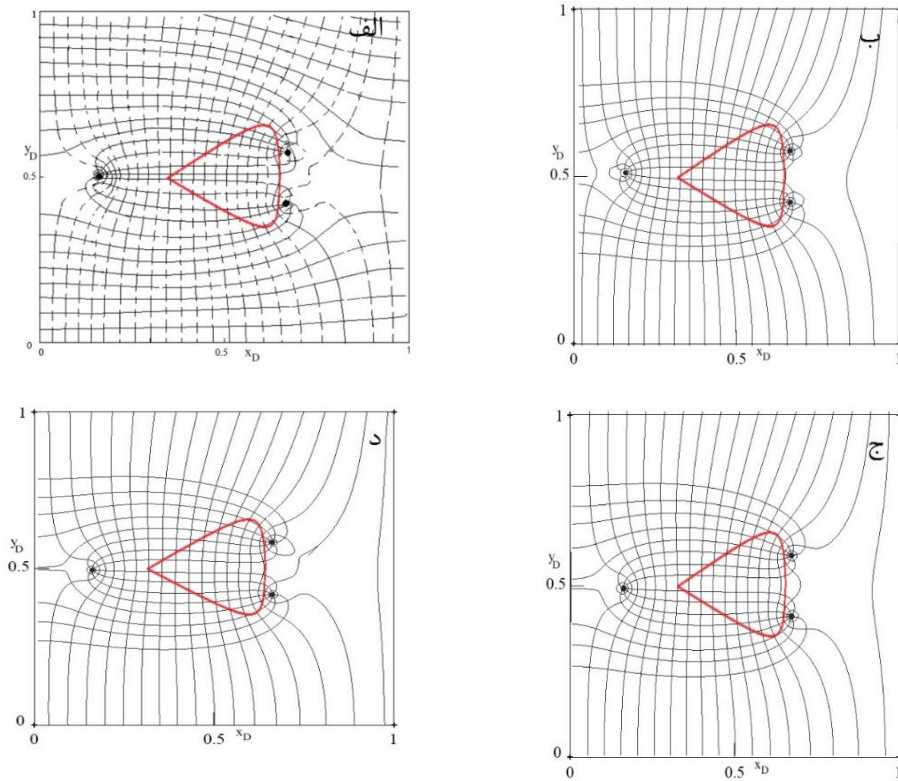
شکل ۵. حوضه آبیگیر شبیه سازی شده در مرحله دوم با مدل های تحلیلی (الف) و عددی (ب، ج و د)، چاه شرقی چاه تغذیه و دو چاه دیگر چاه پمپاژ هستند، ابعاد آبخوان: x_D = y_D = 1 \approx 600m
