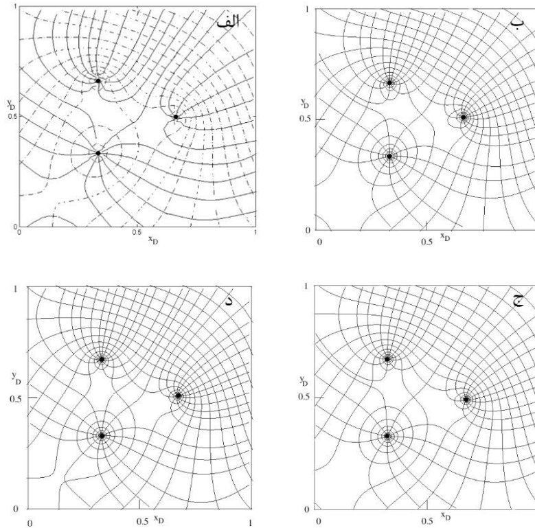
شکل ۳. حوضه آبگیر شبیه سازی شده با مدل های تحلیلی (الف) و عددی (ب، ج و د)، ابعاد آبخوان: x_D=y_D=1 \approx 600m .
