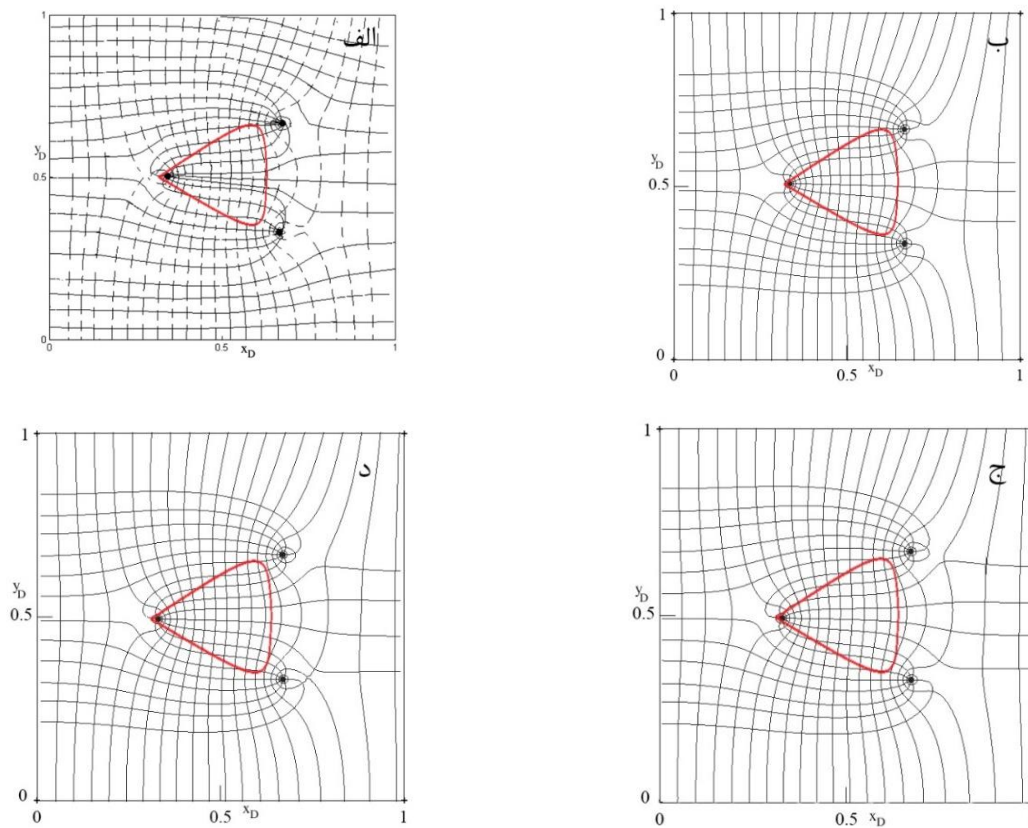
شکل ۴. حوضه آبگیر شبیه سازی شده با مدل های تحلیلی (الف) و عددی (ب، ج و د)، چاه شرقی چاه تغذیه و دو چاه دیگر چاه پمپاژ هستند، ابعاد آبخوان: x_D = y_D = 1 \approx 600m .
