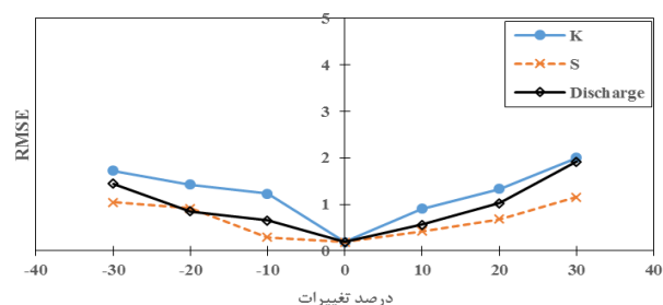
شکل ۱۳. حساسیت مدل نسبت به هدایت هیدرولیکی (K)، آبدهی ویژه (S) و تخلیه آب زیرزمینی (Discharge)
