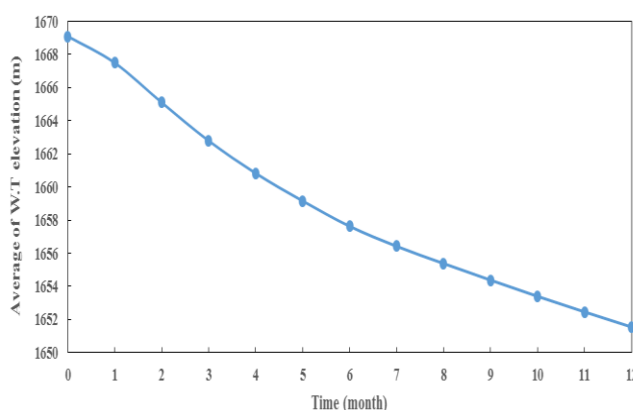
شکل ۱۷. متوسط روند تغییرات سطح ایستابی محدوده پیت معدن
