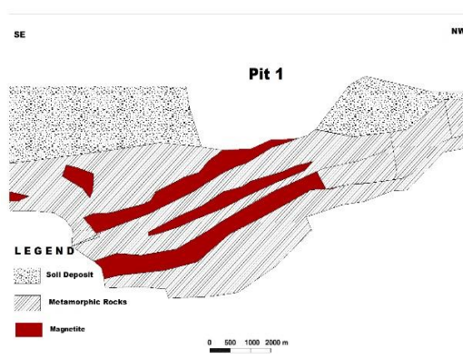
شکل ۴. نیم‌رخ زمین‌شناسی از محدوده‌ی پیت معدن
