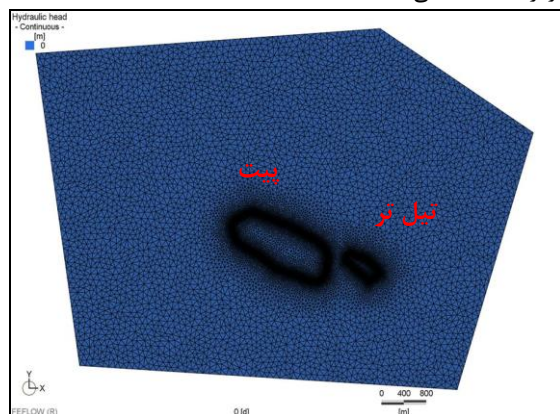
شکل ۶. شبکه‌بندی عناصر محدود در محیط FEFLOW
