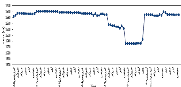
شکل ۵. هیدروگراف واحد آب زیرزمینی محدوده‌ی معدن در بازه زمانی ۱۳۸۵-۹۲
