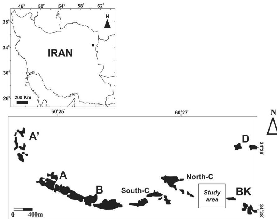
شکل ۱. موقعیت جغرافیایی معدن سنگان در شمال شرق ایران و نمایش موقعیت توده‌های مگنتیتی از غرب به شرق همراه با موقعیت منطقه مورد مطالعه
