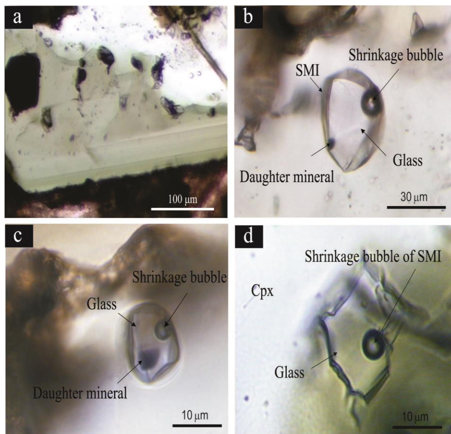
شکل ۳. تصویر میکروسکوپی از آنکلوژیون های مذاب سیلیکاته در میزبان کلینوپروکسن (a). در شرایط درجه حرارت اتاق، حاوی فازهای مختلف می باشند. در این تصاویر آنکلوژیون های مذاب به صورت شکل های تقریباً منظم (b) تا انواع نامنظم (d) تا ابعاد ۵۰ میکرومتر قابل مشاهده اند. همانطور که در تصاویر دیده می شود فاز شیشه < گاز > کانی دختر فازهای اصلی تشکیل دهنده می باشند.
