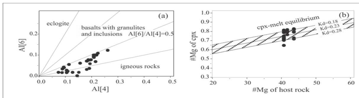
شکل ۷. نمودار Al^6 در مقابل Al^4 کلینوپروکسن های مورد مطالعه، مزره های جداکننده کلینوپروکسن در اکلوتیت، گرانولیت و انکلوزیون بازالت و سنگ های آذرین بر اساس Aoki and Shiba (1973) است. (b) مقدار \#Mg محاسبه شده از کانی کلینوپروکسن در مقابل \#Mg از سنگ میزبان ( 100 * Mg/Mg + Fe^{+2} ) لامپروفیرهای رشته کوه سلوات. محدوده هاشور خورده بیانگر محدوده تعادلی کلینوپروکسن و ترکیب میزبان است ( FeO = 0.85 * Fe_2O_3 ). مقدار K_d ( K_d_{min/liq}^{Fe/Mg} ) بر گرفته از Toplis and Carroll (1995) است.
