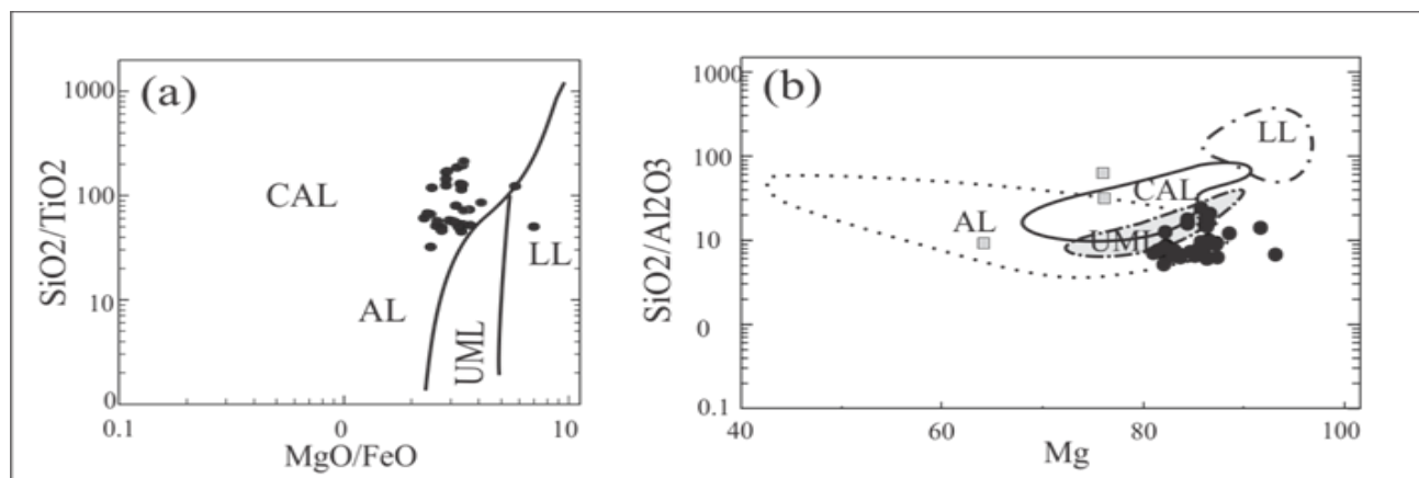
شکل ۹. نمودارهای دو تایی نسبت های SiO 2 /TiO 2 در مقابل MgO/FeO (a) و SiO 2 /Al 2 O 3 در مقابل Mg (b) در کلینوپیروکسن های لامپروفیرهای رشته کوه سلوات. در این نمودارها در محدوده های انواع مختلف لامپروفیر بر اساس (Rock, 1991) است.
