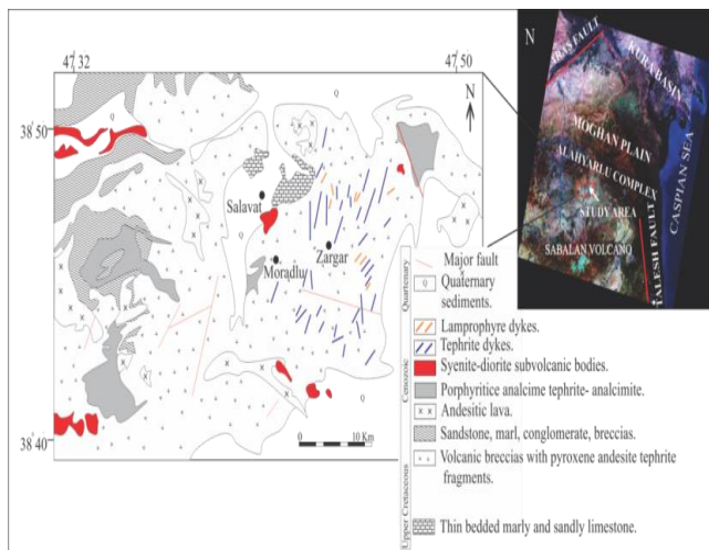
شکل ۱. موقعیت نقشه زمین شناسی ساده از محدوده مورد مطالعه برگرفته از نقشه زمین شناسی ۱:۱۰۰۰۰۰ لاهورد با تعبیرات از (Babakhani et al., 1990) در این نقشه موقعیت دایک های لامپروفیری نسبت به سایر واحدهای سنگی در محدوده مورد مطالعه مشخص شده است.
