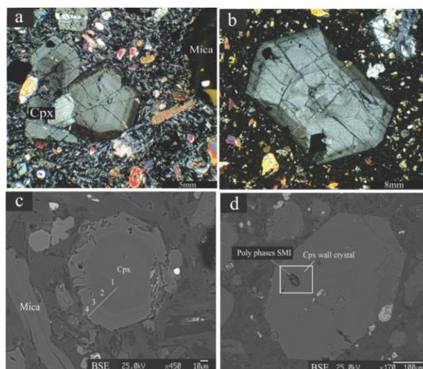
شکل ۲. تصاویر میکروسکوپی (a,b) و بک اسکتر (c,d) از فنوکریست های کلینوپیروکسن در لامپروفیرهای رشته کوه سلوات. در این تصاویر پهنه بندی شیمیایی نوسانی (a,c) و ساعت شنی (b) در فنوکریست کلینوپیروکسن به خوبی قابل تشخیص می باشد. در تصاویر بک اسکتر (c) پهنه بندی شیمیایی نوسانی با تغییر رنگ تیره و روشن با تغییر تمرکز Fe^{+2} , Ca, Al و Ti است، درحالیکه محدوده های تیره بیانگر غنی شدگی در Mg و Si می باشند. حضور انکلوژیون های مذاب چند فاز نیز از مشخصات اصلی این کانی ها است (d).
