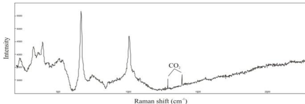
شکل ۴. اسپکتروگراف نمونه از کانی کلینوپیروکسن میزبان آنکلوژیون های مذاب، پیک های CO 2 مربوط به فاز گازی در شرایط دمایی آزمایشگاهی است.
