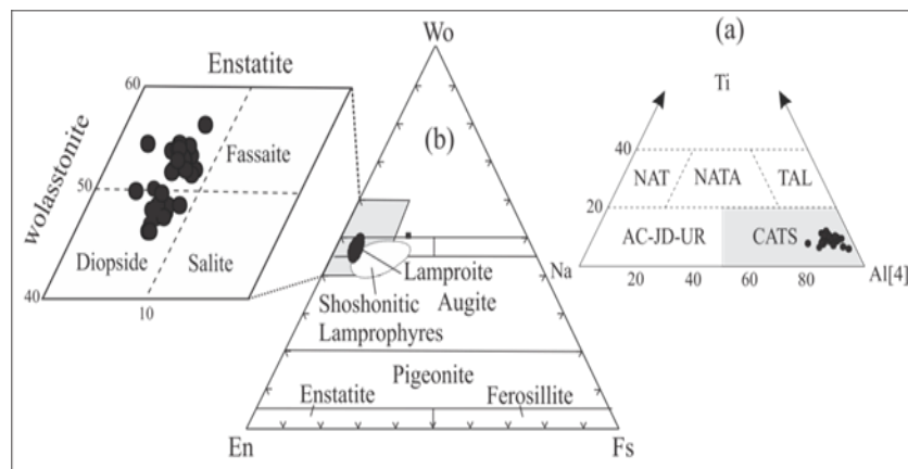
شکل ۵. ترکیب دیوپسیدی فنوکریست های کلینوپیروکسن در لامپروفیرهای رشته کوه سلوات، در نمودار سه تایی [4] Ti-Na-Al (a) (after Papike et al. 1974) NAT-NaTi 0.5 R 0.5 +2Si 2 O 6 ; NATAL-NaTiSiAlO 6 ; TAL-CaTiAl 2 O 6 ; CATS-CaAlAlSiO 6 and نوشتارهای اختصاری به شرح زیر می باشند: CaFeAlSiO 6 ; Ac-NaFeSi 2 O 6 ; JD-NaAlSi 2 O 6 ; UR-NaCrSi 2 O 6 در نمودار سه تایی Ca-Mg-Fe (b) (Morimoto et al., 1989) محدوده های ترکیب کانی کلینوپیروکسن در انواع لامپروفیرهای شوشونیتی و لامپروفیتی (Rock, 1991) به منظور مقایسه مشخص شده اند.
