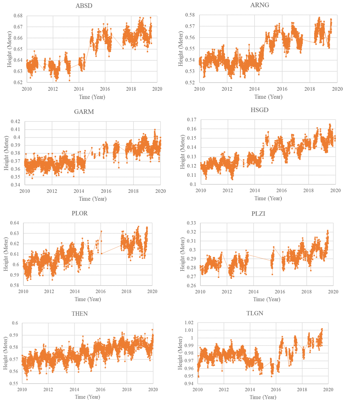
شکل ۵- سری‌های زمانی مربوط تغییرات ارتفاعی ایستگاه‌های IPGN موجود در پهنه ساختاری شمال تهران و نواحی پیرامون آن. تمامی داده‌ها بیانگر بالآمدگی پوسته‌ای ناشی از وجود یک رژیم زمین‌ساختی با مؤلفه فشارشی در منطقه هستند. کم‌ترین نرخ تغییرات ارتفاعی در ایستگاه تهران (TEHN) و بیش‌ترین آن در ایستگاه طالقان (TLGN) مشاهده می‌شود.
