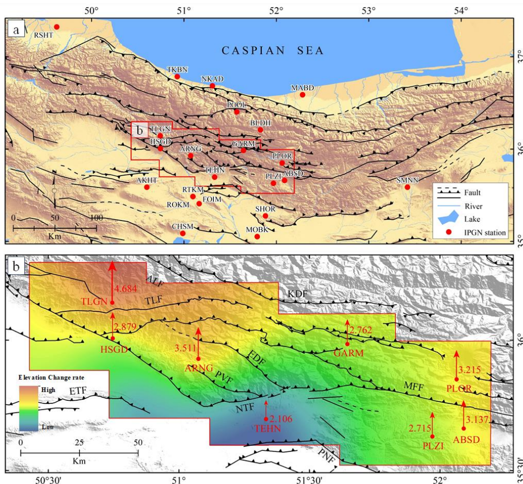
شکل ۴- (a) موقعیت ایستگاه‌های IPGN شمال ایران بر روی مدل ارتفاعی رقومی که بر پایه تصاویر SRTM تهیه شده است. کادر قرمز رنگ موقعیت شکل (b) را نشان می‌دهد، و (b) نقشه نرخ تغییرات ارتفاعی ایستگاه‌های مختلف IPGN بر روی مدل ارتفاعی رقومی.
