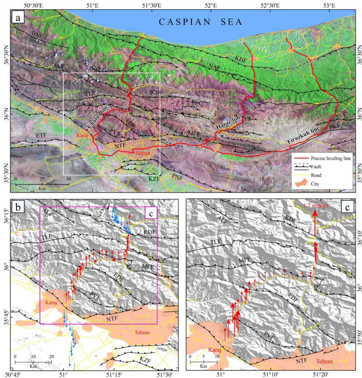
شکل ۶- (a) تصویر ماهواره‌ای Mr.SID البرز مرکزی همراه با نمایش جاده‌های چالوس، هراز و فیروزکوه (خطوط قرمز رنگ) که دارای ایستگاه‌های ترازبایی دقیق در طول خود هستند. در این بین، جاده چالوس از قسمت‌های میانی منطقه پهنا ساختاری شمال تهران عبور می‌کند. کادر سفید رنگ موقعیت شکل (b) را نشان می‌دهد، (b) پیاده سازی ایستگاه‌های ترازبایی دقیق بر روی مدل ارتفاعی رقومی که بر پایه تصاویر SRTM تهیه شده است. پیکان‌های قرمز و آبی بدون رعایت مقیاس، به ترتیب بالآمدگی و فرونشست را در محل ایستگاه‌های ترازبایی نشان می‌دهند. کادر بنفش رنگ بیانگر موقعیت شکل (c) می‌باشد، و (c) نمایش نرخ بالآمدگی محاسبه شده در ایستگاه‌های ترازبایی دقیق در حد فاصل گسل‌های شمال تهران و کندوان. کوتاه‌نوشت‌ها مشابه با شکل ۱.
