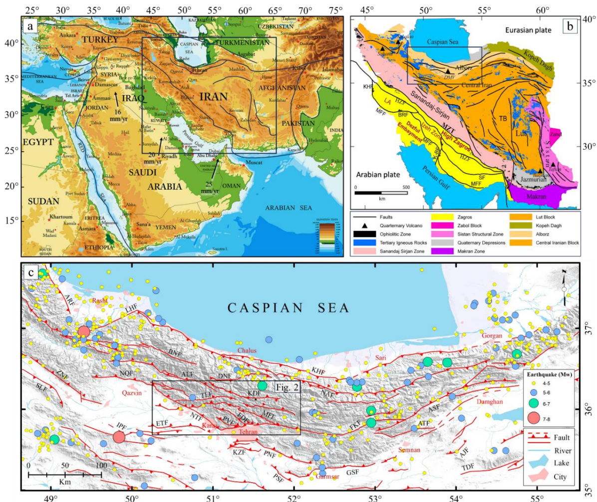
شکل ۱- موقعیت جغرافیایی و زمین‌ساختی محدوده مورد مطالعه. (a) مدل ارتفاعی رقومی منطقه خاور میانه که بر پایه تصاویر SRTM تهیه شده است. خطوط و کادر سیاه رنگ به ترتیب گسل‌های اصلی و موقعیت شکل (b) را نشان می‌دهند، (b) پهنه‌های ساختاری- رسوبی ایران (برگرفته از تکنیک و قدس، ۲۰۱۷)، کادر سیاه رنگ موقعیت شکل (c) را نشان می‌دهد و (c) نقشه لرزه زمین‌ساخت شمال ایران. زمین‌لرزه‌های دستگاهی منطقه مربوط به سال‌های ۱۹۰۰ تا ۲۰۲۴ (برگرفته از سازمان زمین‌شناسی ایالات متحده آمریکا). کادر سیاه رنگ موقعیت شکل ۲ را نشان می‌دهد. کوته‌نوشت‌ها: NTF: گسل شمال تهران، PVF: گسل پورکان- وردیج، EDF: گسل امام زاده داوود، MFF: گسل مشا- فشم، TLF: گسل طالقان، KDF: گسل کندوان، DNF: گسل دشت نظیر، NAF: گسل شمال البرز، KHF: گسل خزر، BNF: گسل بنان، LHF: گسل لاهیجان، ARF: گسل آستارا، NQF: گسل شمال قزوین، ALF: گسل الموت، ZNF: گسل زنجان، SLF: گسل سلطانیه، IPF: گسل ایپک، ETF: گسل اشتهارد، KZF: گسل کهریزک، PNF: گسل پارچین، PSF: گسل پیشوا، GSF: گسل گرمسار، FKF: گسل فیروزکوه، ASF: گسل آستانه، AJF: گسل انجیلو، TDF: گسل ترود.
