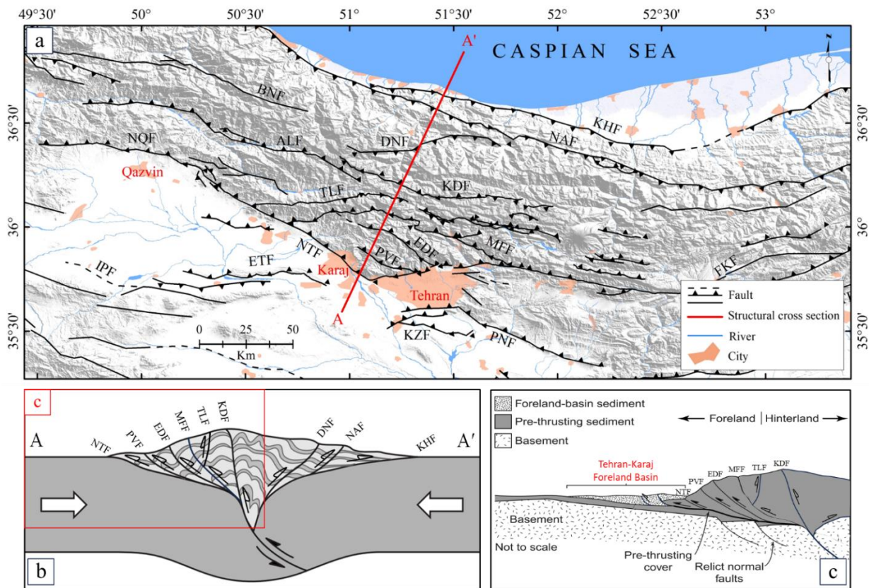
شکل ۳- (a) پیاده‌سازی گسل‌های اصلی منطقه بر روی مدل ارتفاع رقومی. خط قرمز رنگ مسیر بُرش عرضی ساختاری ارائه شده در شکل (b) را نشان می‌دهد، (b) تصویری شماتیک از بُرش عرضی ساختاری البرز مرکزی که بیانگر شکل‌گیری یک گل ساخت مثبت در کمربند البرز مرکزی می‌باشد. کادر قرمز رنگ نشان‌دهنده موقعیت شکل (c) می‌باشد، و (c) مدل ساختاری پیشنهادی برای دامنه جنوبی البرز مرکزی و پهنه ترفاشاری شمال تهران همراه با تشکیل حوضه پیش‌بوم تهران در جنوب این ارتفاعات (بر پایه Pluijm and Marshak, 2004). کوتاه‌نوشت‌ها مشابه با شکل ۱.
