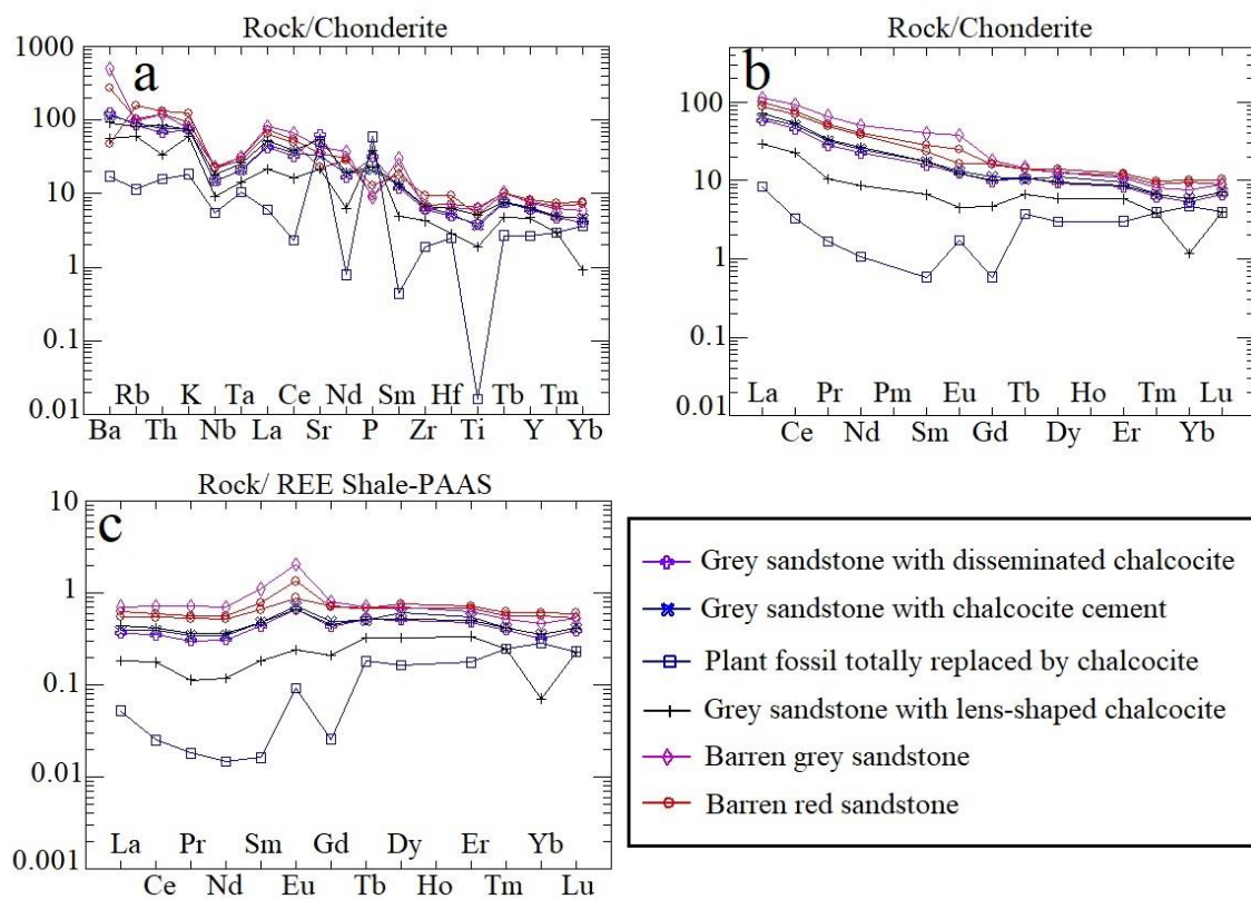
شکل ۸- (a) الگوهای چند عنصری به‌نجارشده نسبت به کندریت (Thompson, 1982) برای نمونه‌های کانه‌دار و ماسه‌سنگ‌های قرمز و خاکستری بدون کانه‌زایی در کانسار حمزه‌لو، (b) الگوهای عناصر کمیاب خاکی به‌نجارشده نسبت به کندریت (Sun and McDonough, 1989) برای نمونه‌های کانه‌دار و ماسه‌سنگ‌های قرمز و خاکستری بدون کانه‌زایی در کانسار حمزه‌لو، (c) الگوهای عناصر کمیاب خاکی به‌نجارشده نسبت به شیل استرالیا (Taylor and McLennan, 1985) برای نمونه‌های کانه‌دار و ماسه‌سنگ‌های قرمز و خاکستری بدون کانه‌زایی در کانسار حمزه‌لو.
