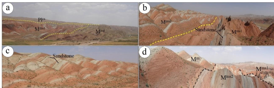
شکل ۳- (a) نمای از واحدهای M^{mg} ، M^{ms1} و Pl^{cs} در منطقه حمزه‌لو (دید به سمت شمال‌خاور)، (b) تناوب مارن‌های قرمز با میان‌لایه‌های ماسه‌سنگ خاکستری واحد M^{ms1} که توسط واحد M^{ms2} پوشیده شده‌اند (دید به سمت شمال‌باختر)، (c) تناوب مارن‌های قرمز و سبز با میان‌لایه‌های ماسه‌سنگی واحد M^{ms2} (دید به سمت باختر)، (d) نمایی از واحدهای مارنی M^m که به‌طور هم‌شیب بر روی واحدهای M^{ms1} و M^{ms2} قرار گرفته است (دید به سمت شمال‌باختر).
