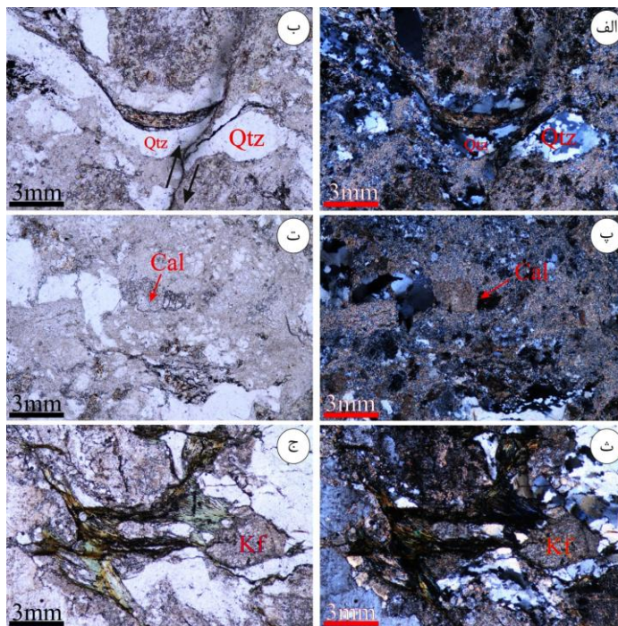
شکل ۴. الف: نمایی از محدوده‌های کلیواژ آناستاموزینگ قطع شده بوسیله ریزگسل معکوس و رفتارهای داکتیل و بریتل کانی‌های کوارتز در خمیره، پهنای میدان دید ۳mm، XPL. ب: PPL. پ: کانی کلسیت با ماکل‌های دگرشکلی تیپ I و II، پهنای میدان دید ۳mm، XPL. ت: PPL. ث: پورفیروکلاست‌های آلکالی فلدسپار همراه با شواهد آلتراسیون و تمرکز کانی‌های بیوتیت و کلریت حاصل از تجزیه بر روی سطح کانی‌ها، پهنای میدان دید ۳mm، XPL. ج: PPL.
