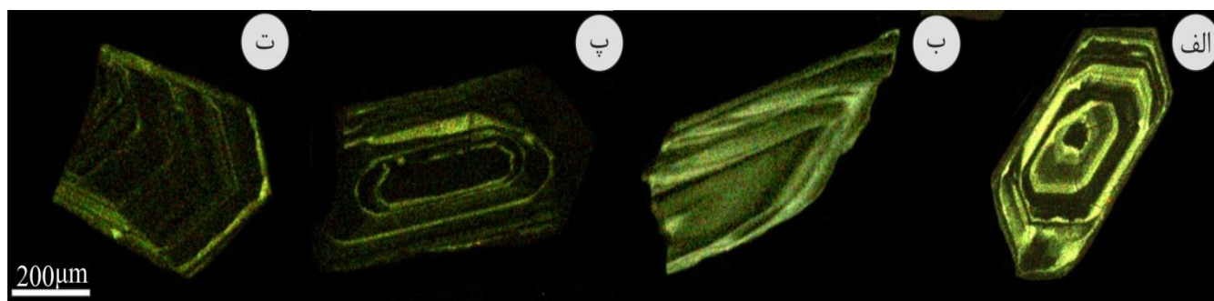
شکل ۵. الف، ب، پ، ت: تصاویر کاتولومینسانس حاصل از دانه‌های زیرکن استخراج شده از گرانیت‌گنایس میلیونیتی جنوب عادگان همراه با زونینگ نوسانی بموازات سطوح منشوری.
