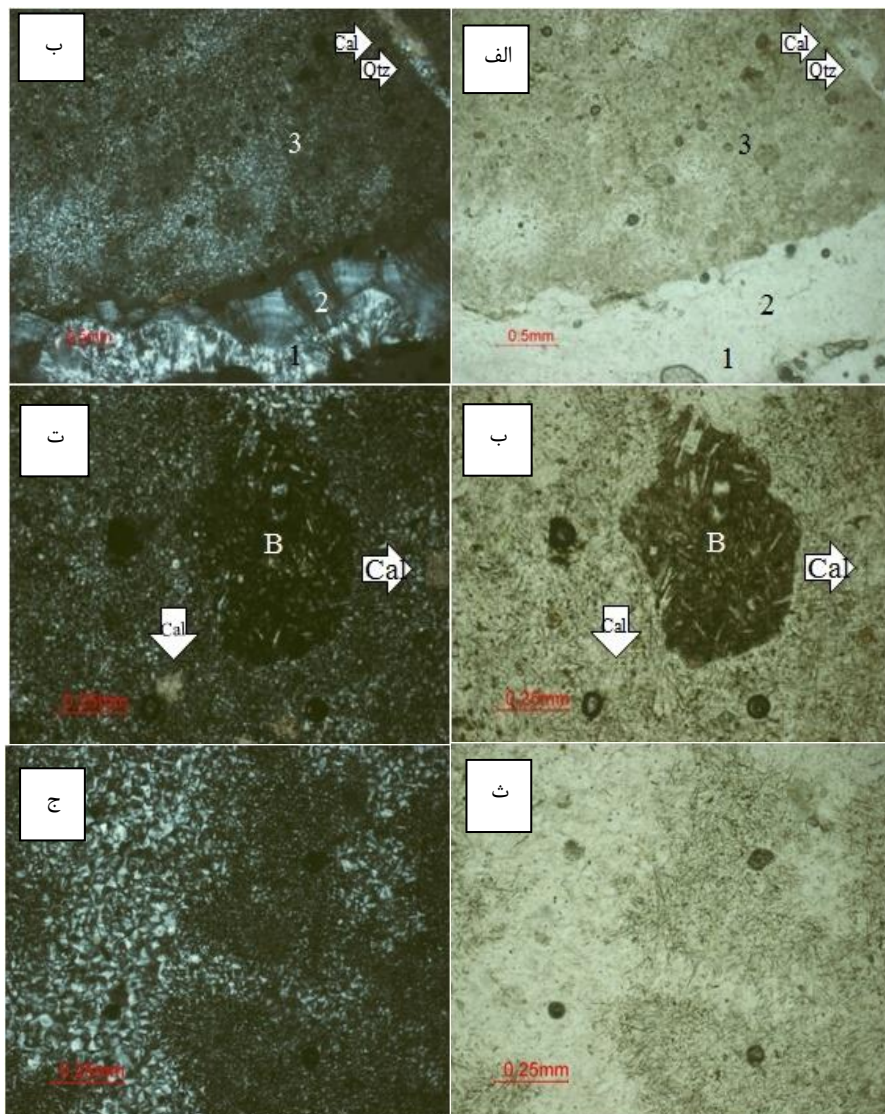
شکل ۸. الف (PPL) و ب (XPL) ۱. بافت واریولیته. ۲. بافت آکسیولیته تا واریولیته. ۳. بافت کریپتوکریستالین. کلسیت و کوارتز پرکننده شکستگی ها. پ (PPL) و ت (XPL) قطعات بازالت و کلسیت موجود در آگات. ث (PPL) و ج (XPL) روتیل های سوزنی موجود در بخش کریپتوکریستالین آگات.
