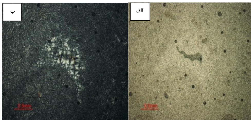
شکل ۴. بافت کریپتوکریستالین که در بعضی قسمت ها به میکروواربولیتی تا میکرواسفرولیتی تغییر یافته است و لکه های اکسید آهن (لکه های قهوه ای در قسمت بالا سمت راست) در الف (نور PPL) و ب (نور XPL)
