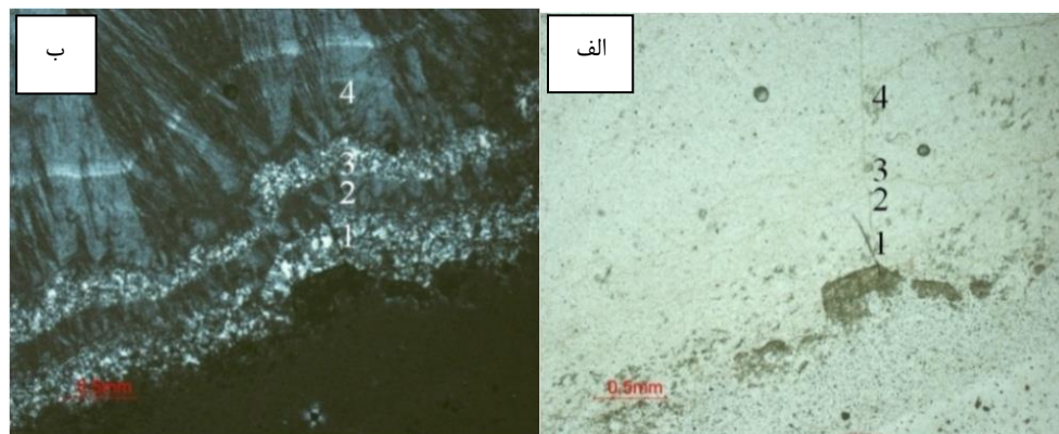
شکل ۶. ۱. بافت میکروگرانولار، ۲. بافت واریولیتی، ۳. بافت میکروگرانولار، ۴. بافت آکسیولیتی تا ماکروواریولیتی در الف (PPL) و ب (XPL)
