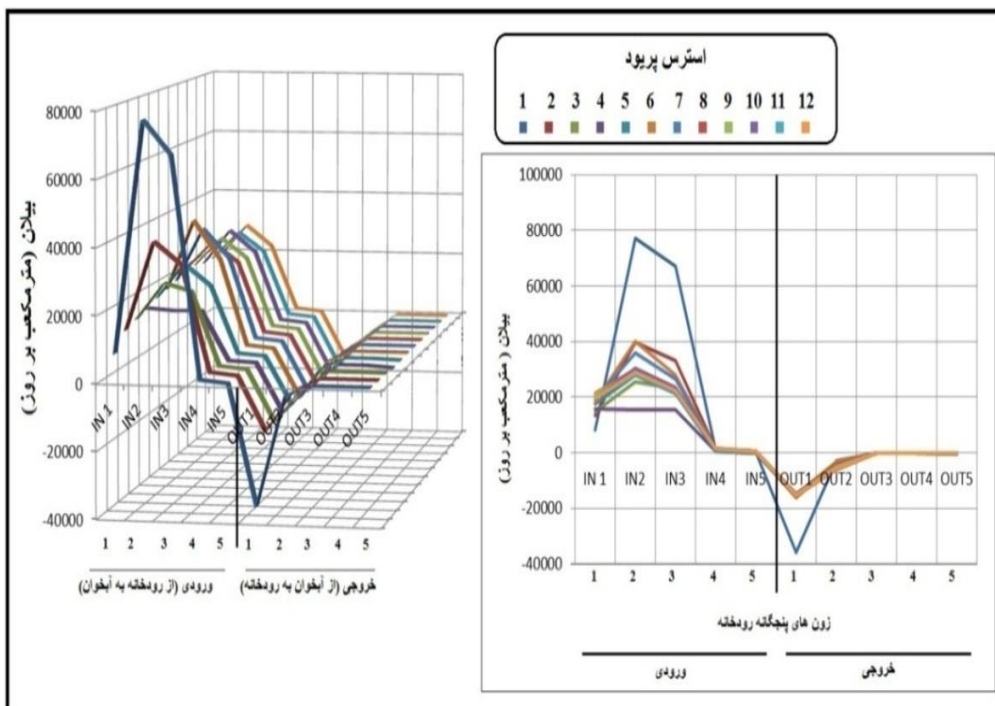
شکل ۱۴. ۱۲ بیلان در مناطق پنجگانه رودخانه در استرس های مختلف در دوره خشکسالی
