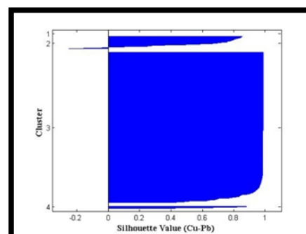
دسته‌بندی با K=4 با مقدار متوسط ۰/۹۲۹۲
