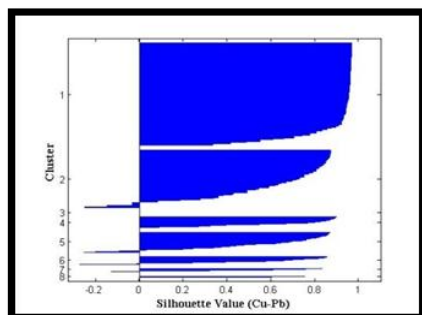
دسته‌بندی با K=8 با مقدار متوسط ۰/۷۴۳۹
