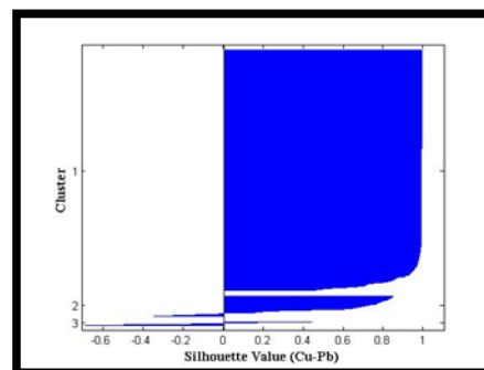
دسته‌بندی با K=3 با مقدار متوسط ۰/۹۱۶۱
