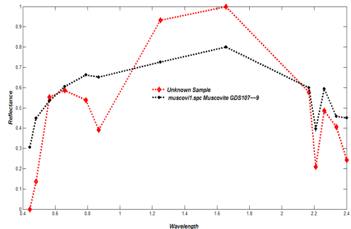
شکل ۹. نتایج اعمال الگوریتم فوق بر روی داده‌های هایپریون محدوده معدن مس دره‌زار. نمودار قرمز مربوط به طیف ناشناس و نمودار مشکی مربوط به طیف کتابخانه‌ای کانی مسکوویت می‌باشد.
