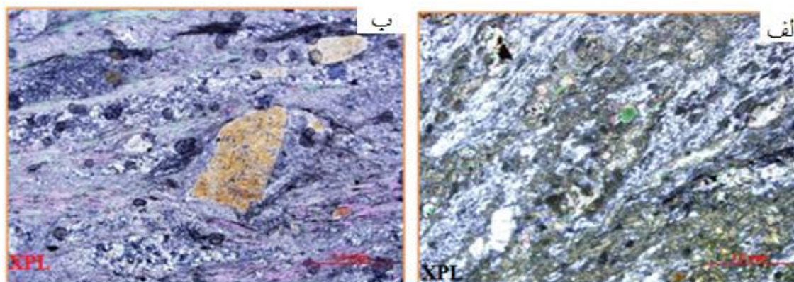
شکل ۳. (الف) باندهای جهت یافته از بیوتیت، موسکوویت به همراه فلدسپات های آلکان و پلاژیوکلاز، در زمینه زمینه کاملاً آهکی کالک شیسست با بافت لپیدوپروفریروولاستی، (ب) نمایی از بافت لپیدوپروفریروولاستی کالک شیسست.
