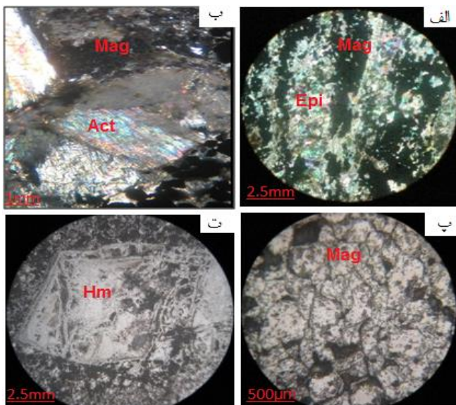
شکل ۶ الف) همرشدی و درگیری میکرونی مگنتیت با اپیدوت، ب) همرشدی مگنتیت با اکتینولیت، پ) نمایی از بلورهای هم بعد نیمه شکل دار مگنتیت همرشد با گانگ، ت) سودومورف هماتیت به جای مگنتیت کاملاً شکل دار.
