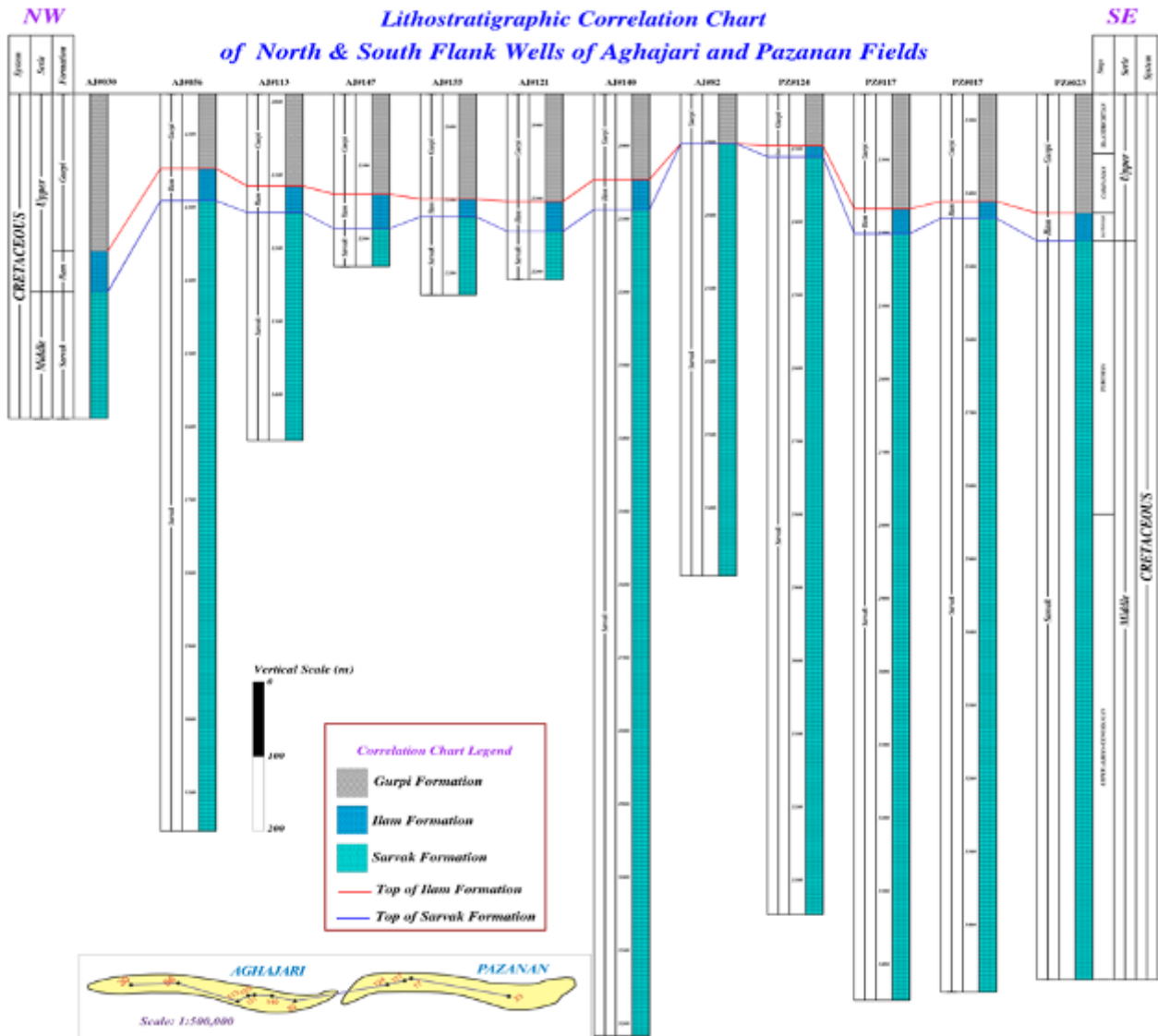
شکل ۱۱. چارت تطابقی (Correlation chart) سنگ چینه ای مربوط به سازند ایلام در میدان آغاجاری و پازنان نشان دهنده محو شدن سازند ایلام در مرز بین دو تاکدیس است.
