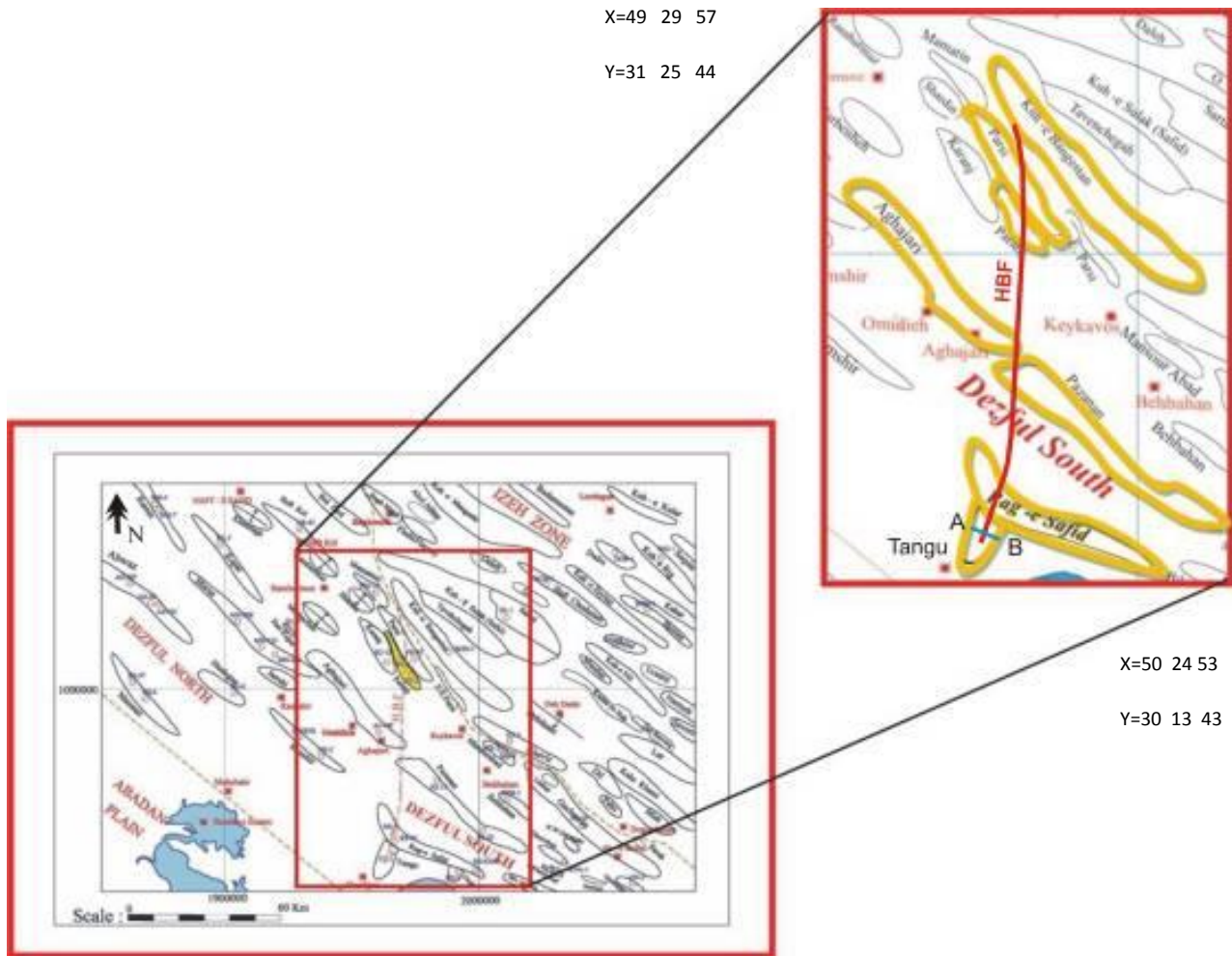
شکل ۱. موقعیت منطقه مورد مطالعه در فرو افتادگی دزفول که میادین مورد نظر در آن با حاشیه ضخیم و رنگی مشخص گردیده اند. خط A-B در میدان تنگو موقعیت پروفیل لرزه ای شکل ۲ را نشان می دهد (سیستم مختصات نقشه مبنا لامبرت می باشد).
