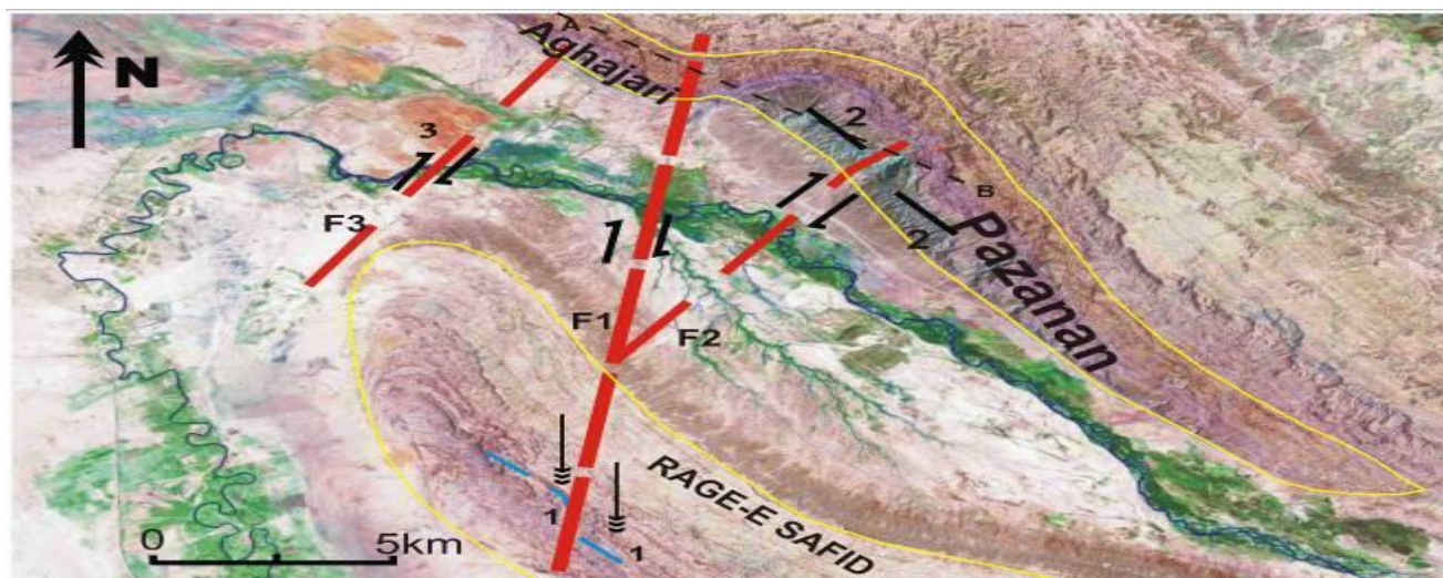
شکل ۶. تصویر ماهواره ای از دماغه شمال غربی میداین رگ سفید و پازنان که نشاندهنده تاثیر حرکات سیستم گسلی هنديجان- بهرگانسر بر این میداین است. خط چین A-B موقعیت پروفیل لرزه ای شکل (۷) را نشان می دهد.
