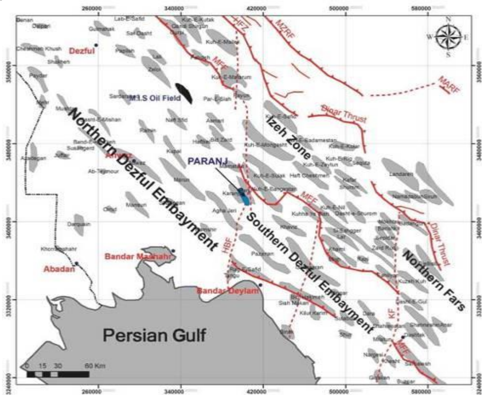
شکل ۱۲. گسل هندیمان - بهرگانسر بر دماغه جنوب شرقی تاقدیس پرنج (رنگ آبی) اثر گذاشته است. HBF=گسل هندیمان- بهرگانسر (اقتباس از: Sherhati, 2005).
