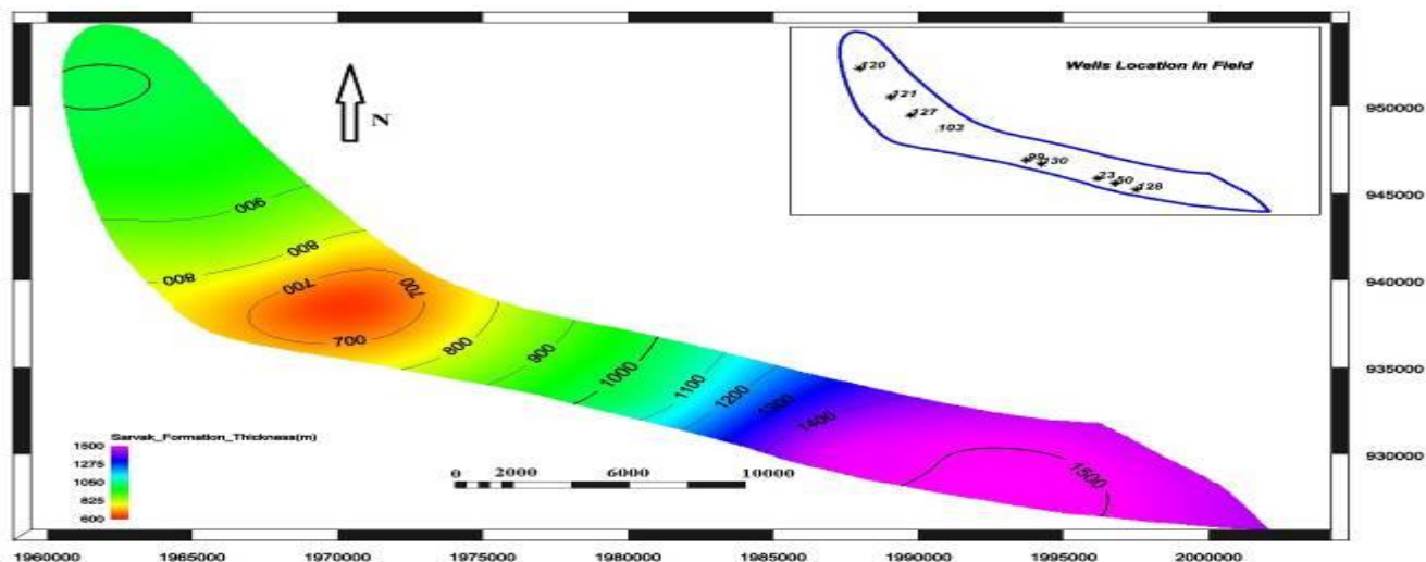
شکل ۵. نقشه هم ضخامت سازند سروک در میدان رگ سفید که نشان می دهد در محل چرخش دهانه شمال غربی ضخامت سازند سروک کمتر است. این مکان در زمان رسوب گذاری این سازند، بر اثر حرکات گسل پی سنگی هنديجان - بهرگانسر بلندتر از قسمت های دیگر میدان بوده و می تواند محل تاثیر بیشتر این گسل باشد.
