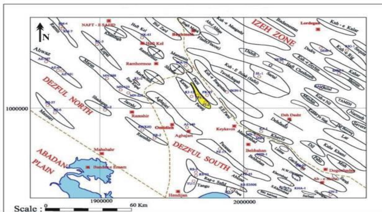
شکل ۱۶. نقشه میداین فرو افتادگی دزفول (انتشار یافته در سال ۸۳ توسط مدیریت اکتشاف) جهت موقعیت میدان پرنج که نشان می دهد گسل هندیمان - بهرگانسر فرو افتادگی دزفول را به دو بخش شمالی و جنوبی تقسیم کرده است. بر اساس این نقشه قبلی گسل هندیمان از مرز میداین آغاچاری و مارون می گذرد.
