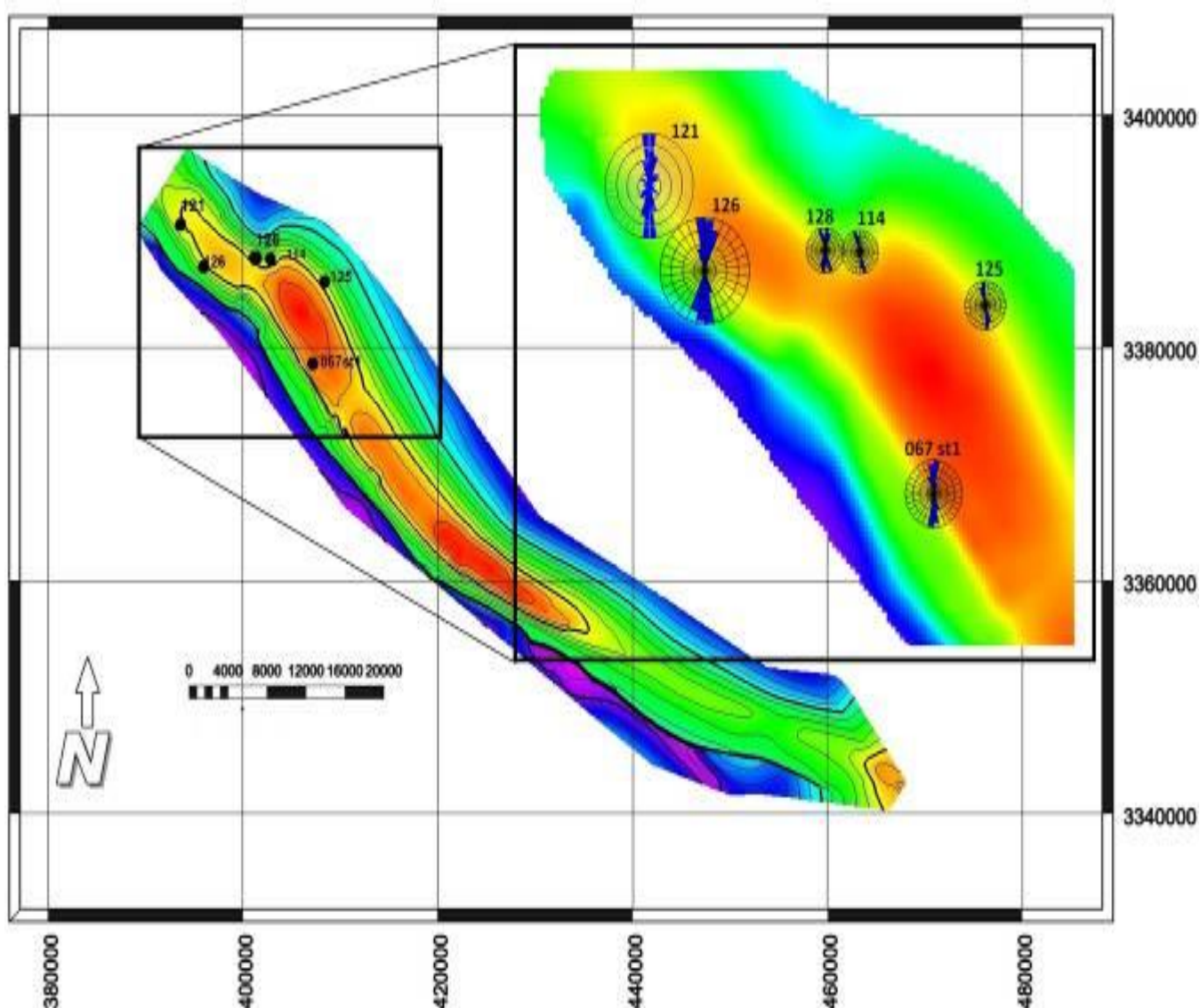
شکل ۸. دیاگرام گل سرخی از شکستگی های با روند N-S در دماغه شمال غربی پازنان - قطر بیشتر دیاگرام گل سرخی در ۲ چاه ۱۲۱ و ۱۲۶ نشان می دهد شکستگی های با روند شمالی تحت تاثیر گسل هندیجان در این دو چاه نسبت به بقیه چاه ها بیشتر می باشد (در این شکل فقط شکستگی های با روند شمالی جهت مقایسه نسبت آنها در چاه های مختلف آورده شده است).
