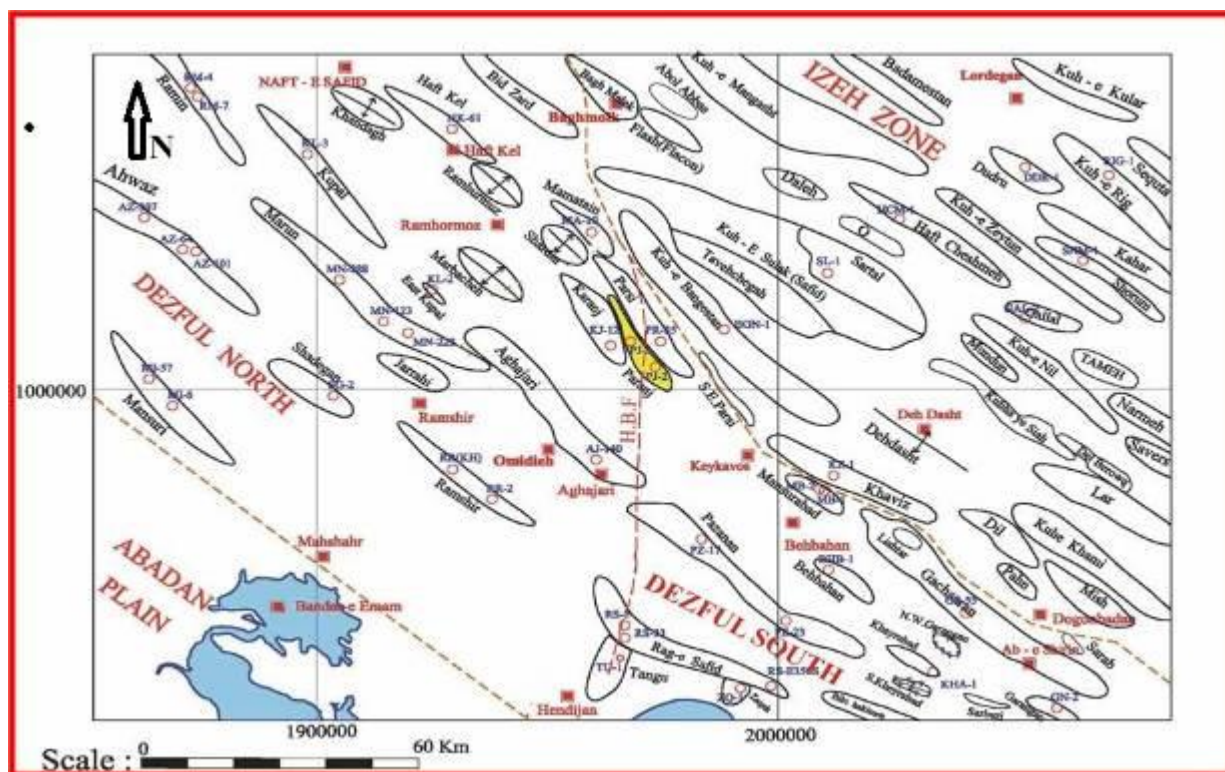
شکل ۱۷. مسیر تصحیح شده گسل هندیدجان - بهرگانسر بر اساس این تحقیق که نشان میدهد این گسل میادین تنگو، رگ سفید، آغاچاری، پازنان پارسی، پرنج و کوه بنگستان را تحت تاثیر قرار داده و برخلاف نقشه بالا از مرز بین میادین آغاچاری و پازنان عبور می کند.
