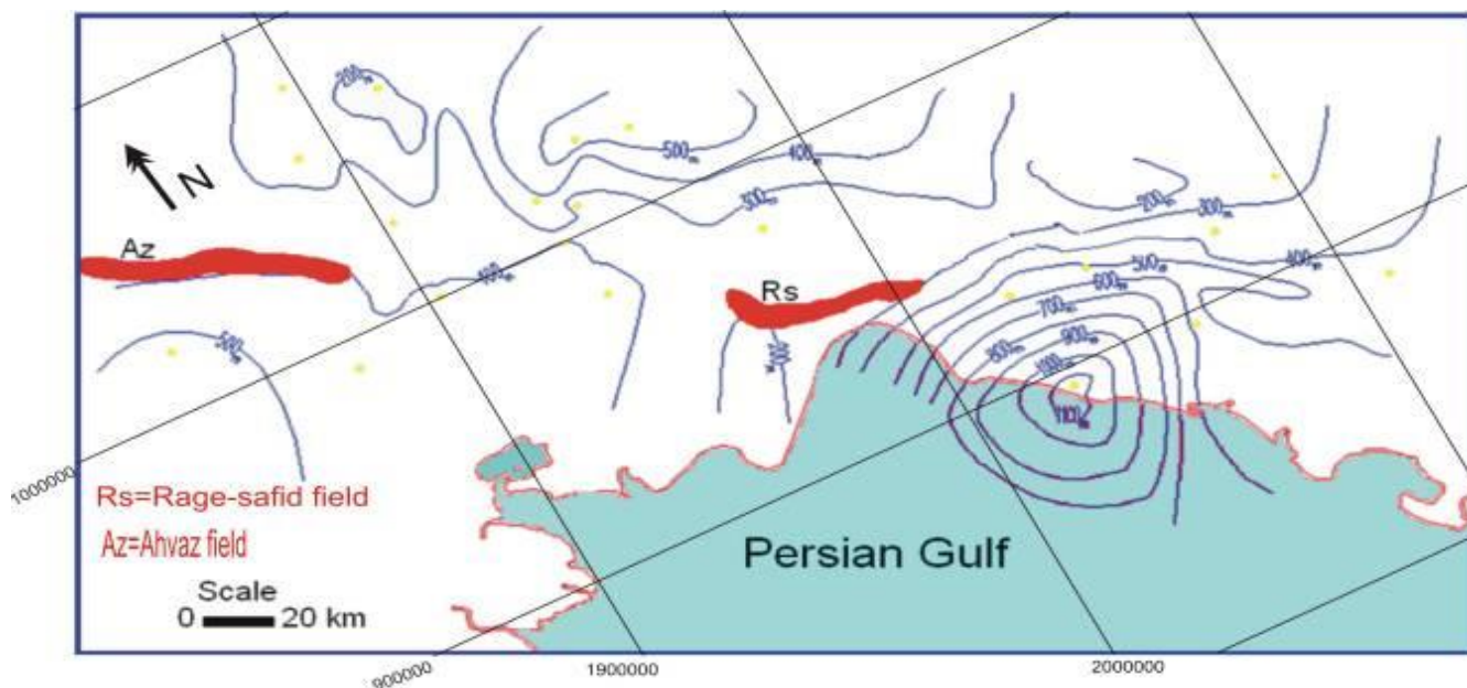
شکل ۴. نقشه هم ضخامت مجموع سازندهای پابده و گوربی در فروافتادگی دزفول (به میزان ضخامت این سازندها در میداین اهواز (AZ) و رگ سفید (RS) توجه شود)
