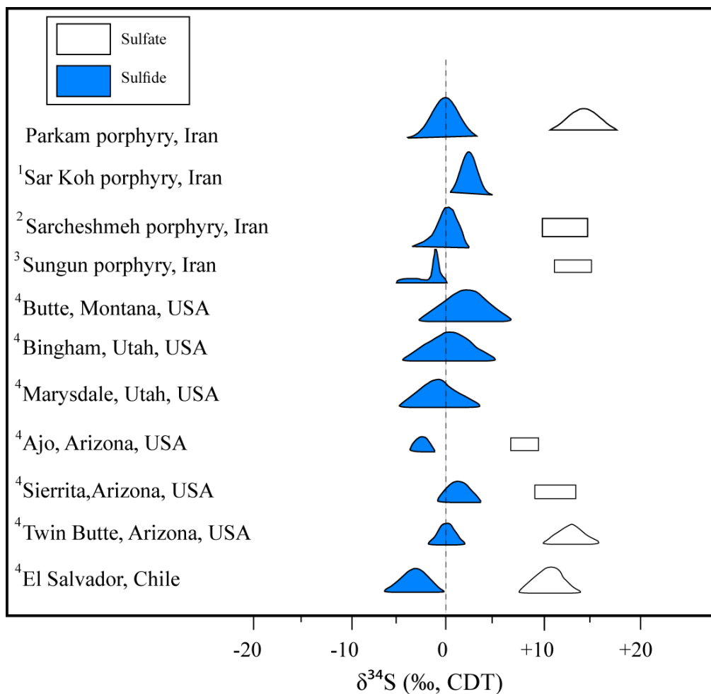
شکل ۹. مقایسه دامنه تغییرات مقادیر \delta^{34}\text{S} کانی های سولفیدی و سولفاتی کانسار مس پورفیری پرکام با بعضی از کانسارهای مس پورفیری ایران و جهان. Ohmoto and Rye (2003), Calagari (2003), ۳ (1979) معانی جو و همکاران (۱۳۹۱)، ۱ Nourali and Mirnejad (2012).
